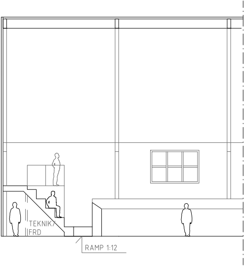
SEKTION B-B
