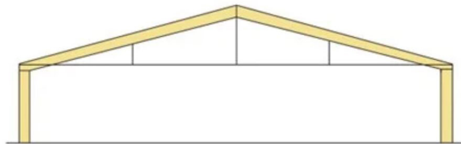
Dragbandstakstol på pelare 15 – 50 m.
